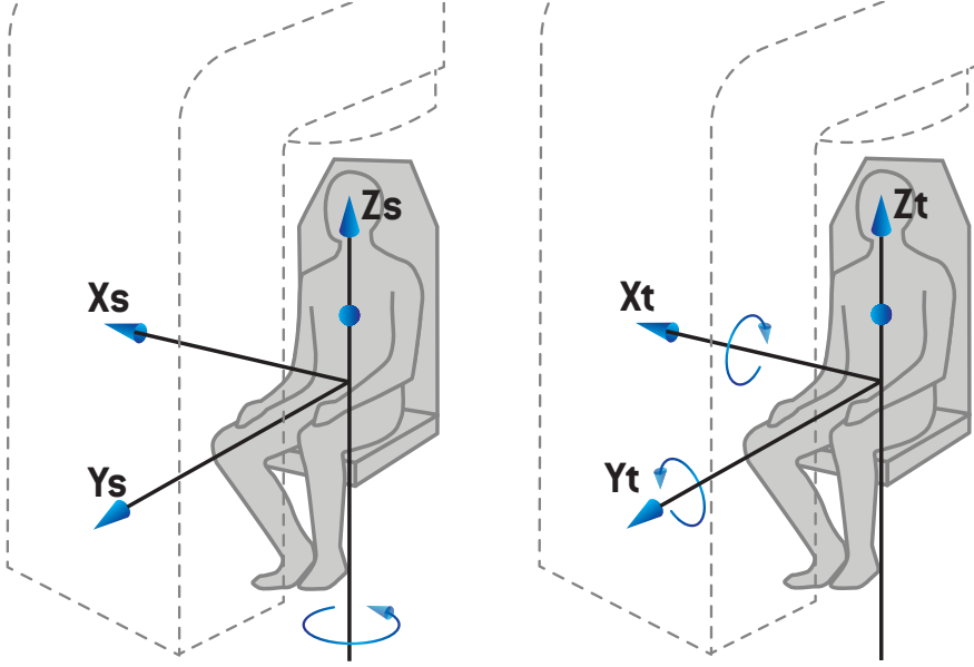
Resim 9. Oturarak tedavi pozisyonu - Dönme açısı için hasta destek koordinat sistemi ve yükselme ve dönüş açıları için masa üstü koordinat sistemi
