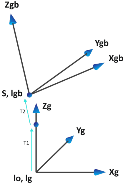
Resim 8. I_o = İzomerkez, S = Kaynak, gb = Gimbal koordinat sistemi, g = Gantry koordinat sistemi, T_1 = birinci öteleme ve T_2 = ikinci öteleme olmak üzere kaynak konumunun çizimi.
